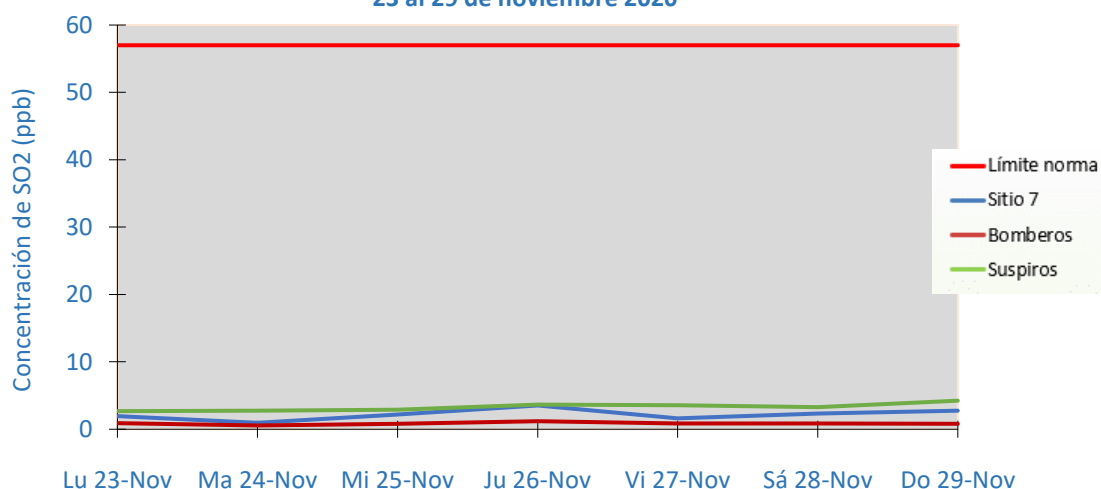
SO 2 - Promedio 24 hrs. - Todas las Estaciones 23 al 29 de noviembre 2020
