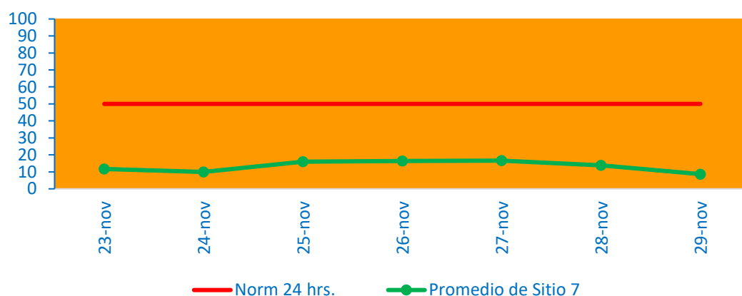
Material Particulado MP 2,5 Promedio 24 hrs.
