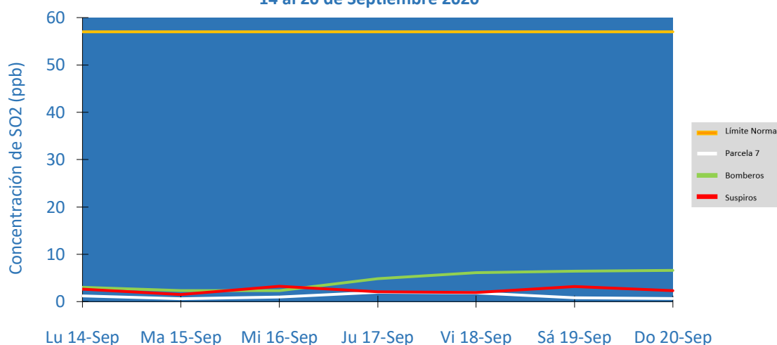
SO 2 - Promedio 24 hrs. - Todas las Estaciones 14 al 20 de Septiembre 2020
