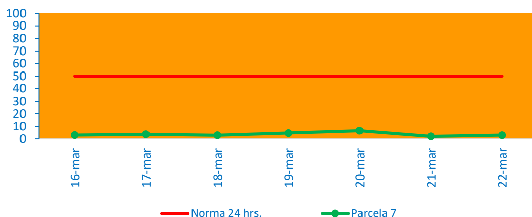
Material Particulado MP 2,5 Promedio 24 hrs. Marzo 2020
